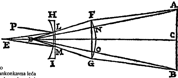
Slika 12. Kombinacija plankonkavne i plankonveksne leće radi motrenja posve udaljenih predmeta: de Dominisova teorijska priprema za izlaganje o dalekozoru. De Dominis, De radiis , p. 35.
